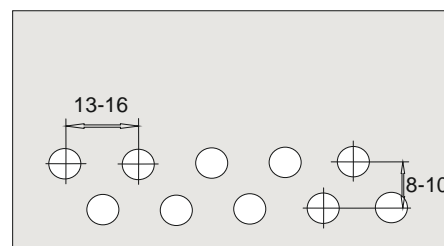
Bohrlochanordnung
