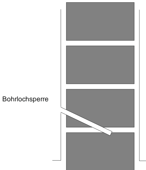
Mauerquerschnitt
